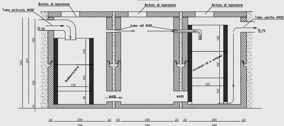
SEZIONE A-A
